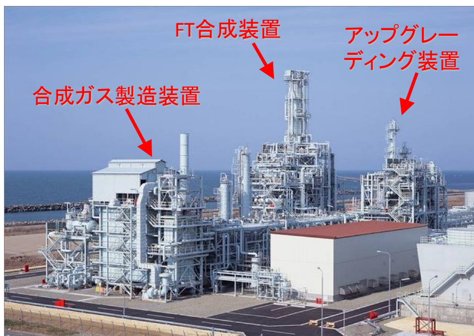
図 3 GTL 実証プラント (500BPD)
